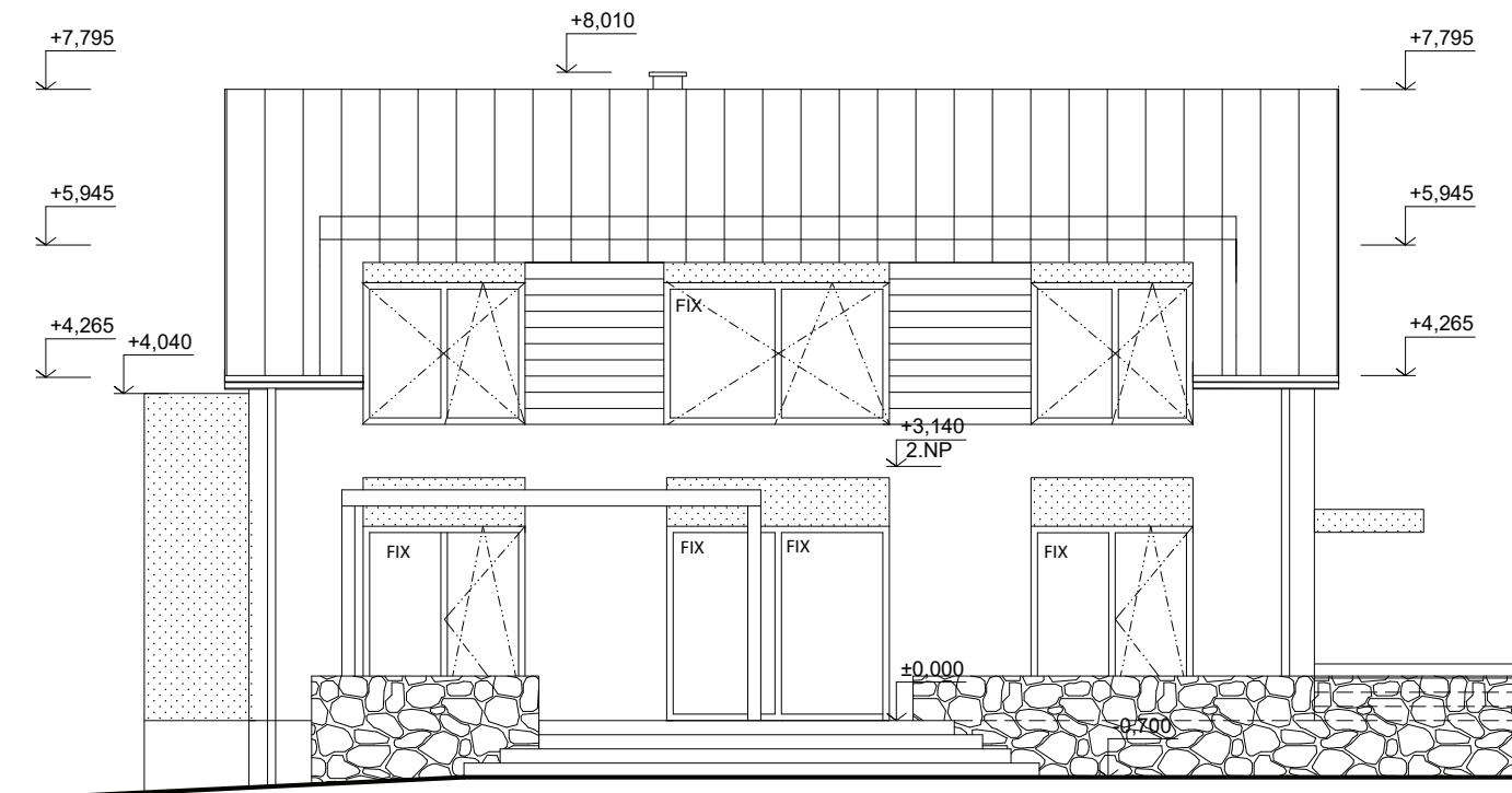
JIŽNÍ POHLED
