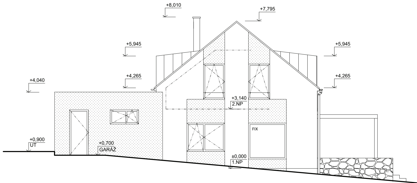
ZÁPADNÍ POHLED
