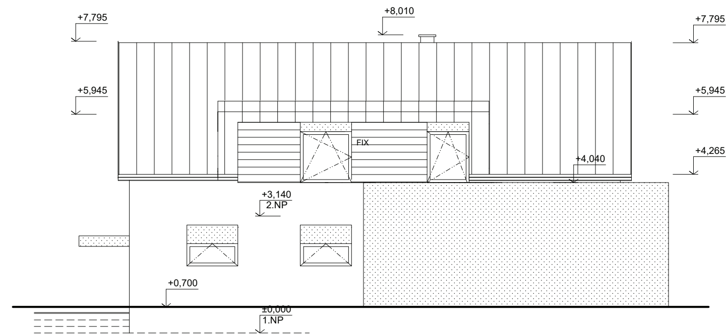
SEVERNÍ POHLED
