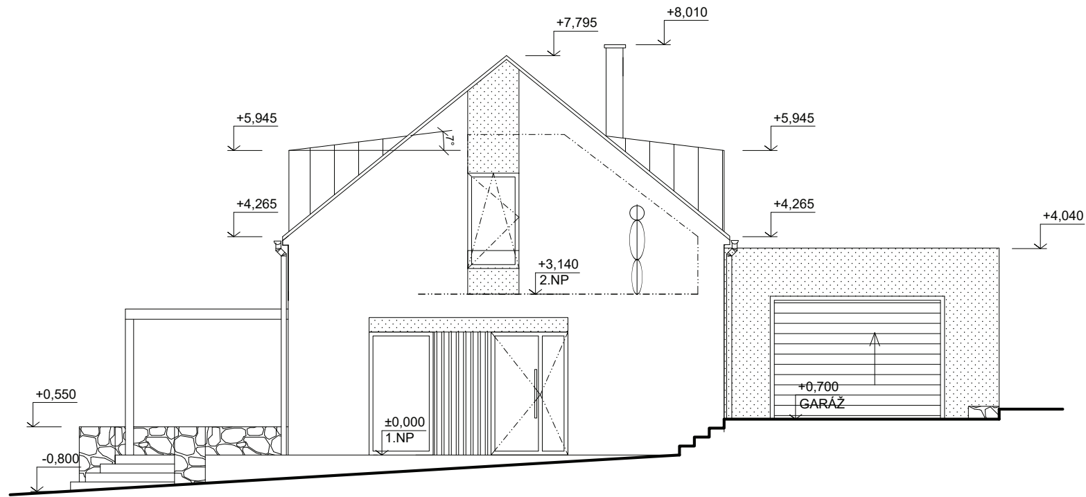
VÝCHODNÍ POHLED
